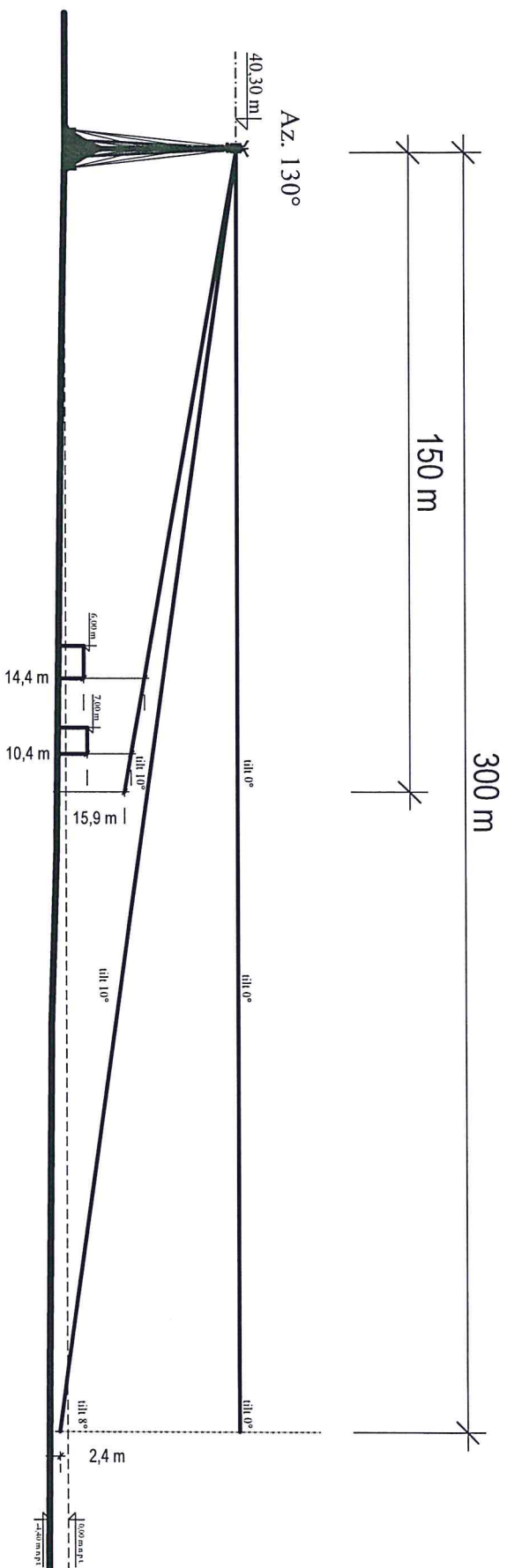
Rys. 3. Rzut pionowy osi głównej wiązki promieniowania na azymucie 130^\circ w odległości do 150 i 300 metrów od środka elektrycznego anteny sektorowej dla tiltów 0^\circ , 8^\circ oraz 10^\circ .
